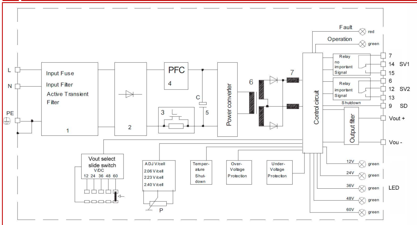
1) Active Transient Filter 2) Rectifier 3) Inrush Current Limiter 4) PFC 5) Load Capacitor 6) Transformer 7) Storage Choke
